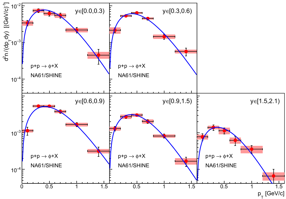
(a) 158 GeV/c
