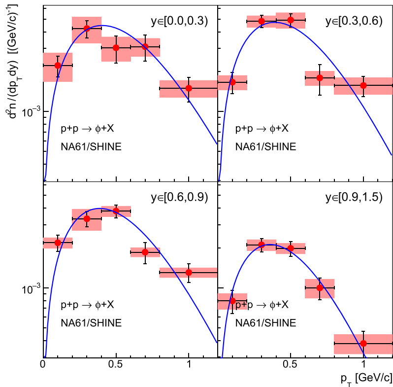
(b) 80 GeV/c
