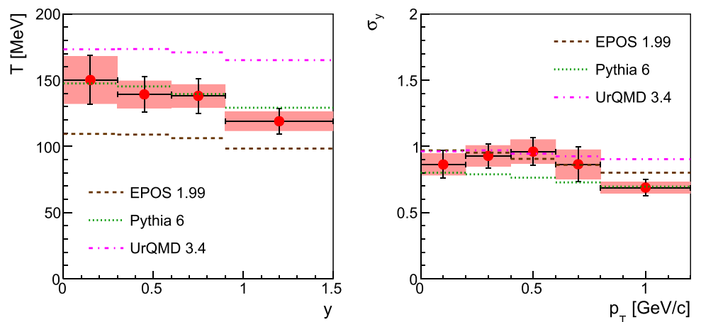
(b) 80 GeV/c
