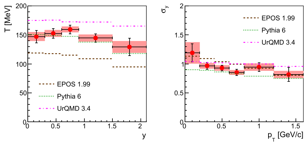
(a) 158 GeV/c
